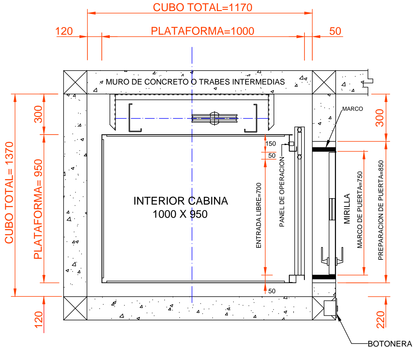
ELEVADOR UNIFAMILIAR HIDRAULICO CHS-210-0.20 TIPO HR
